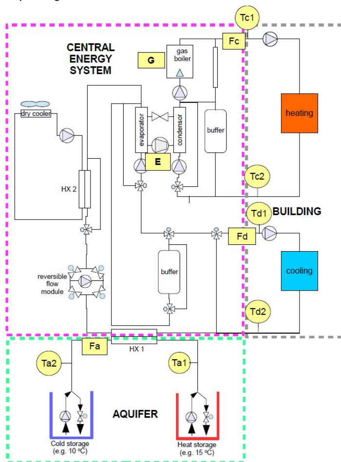
Figuur 3.6 Prinsipeschema van het Rucphen gemeentekantoor
