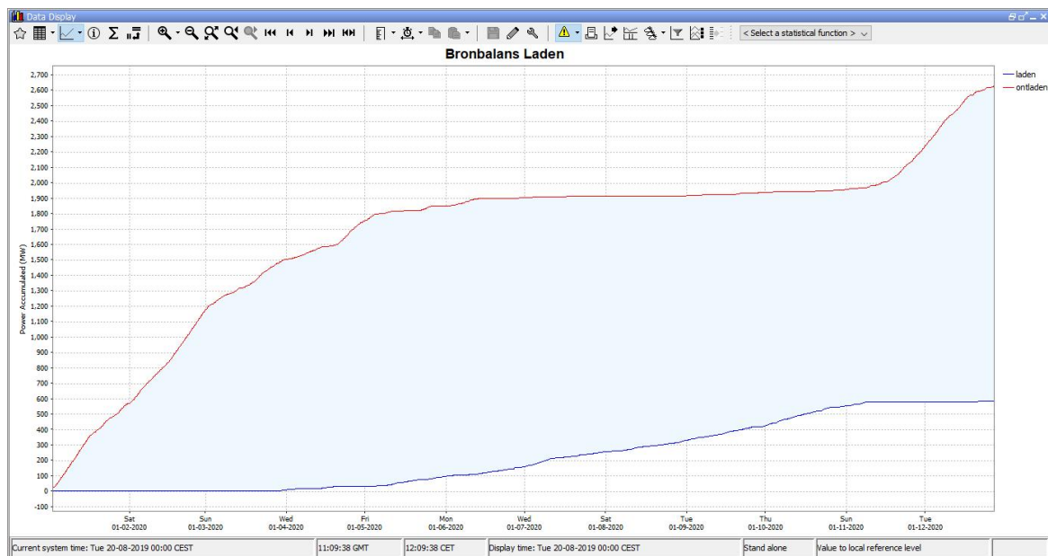
Figuur 3.2 Gesimuleerde voorspelde bronbalans grafiek uit MoBaMo-BES Westraven, waarin de bekende jaarlijkse onbalans tussen kouden laden en ontladen wordt geïllustreerd
