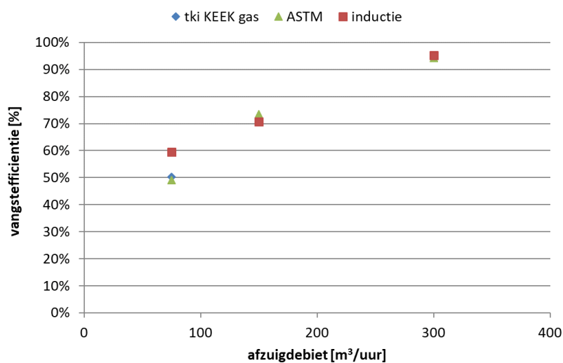
Figuur 22 T-shape: vergelijking vangst efficiëntie van 3 bepalingmethode onder de condities in Tabel 8.
