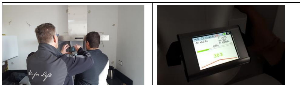
Figuur 14 meting afzuigdebiet motorloze afzuigkap op 23 februari 2018.
