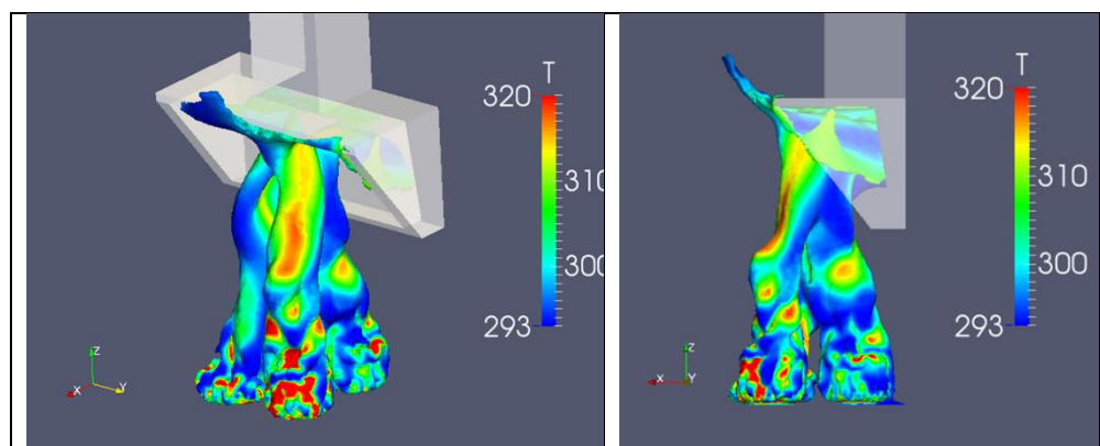
'Horeca' afzuigkap, berekende afzuigefficiency 78% bij 300 m 3 /uur, links vooraanzicht en rechts zijaanzicht.
