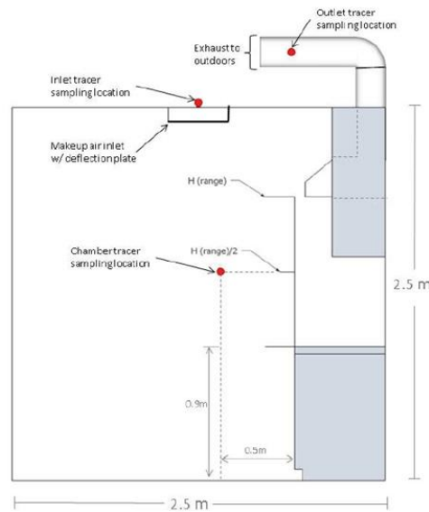
Figuur 18 dwarsdoorsnede van ASTM testkamer, links en rechts van de afzuigkap zijn bovenkastjes.
