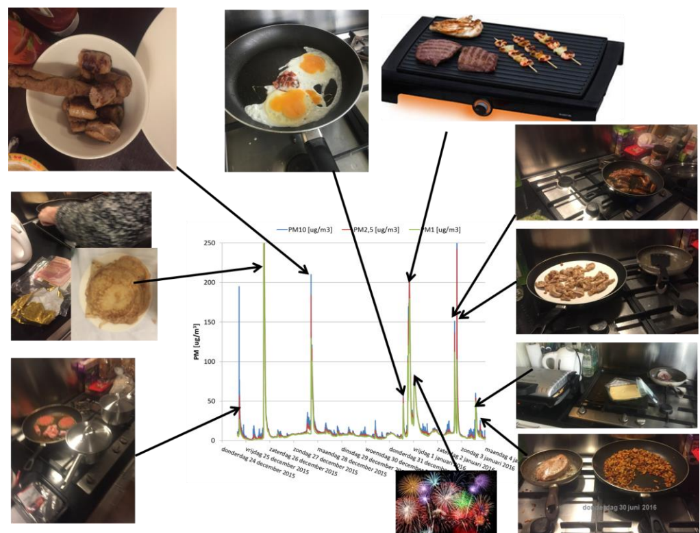
Figuur 1 de in een nieuwbouw woning met motorloze afzuigkap gemeten fijnstof concentraties zijn vooral gerelateerd aan kookactiviteiten 1 .
