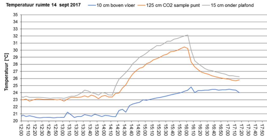
Figuur 24 ASTM meting X-kap 60°, temperatuur in proefkamer voor de kookplaat op drie verschillende hoogten, 14 september 2017: 14.35 uur 150 m 3 /uur, 16.04 uur 300 m 3 /uur.
