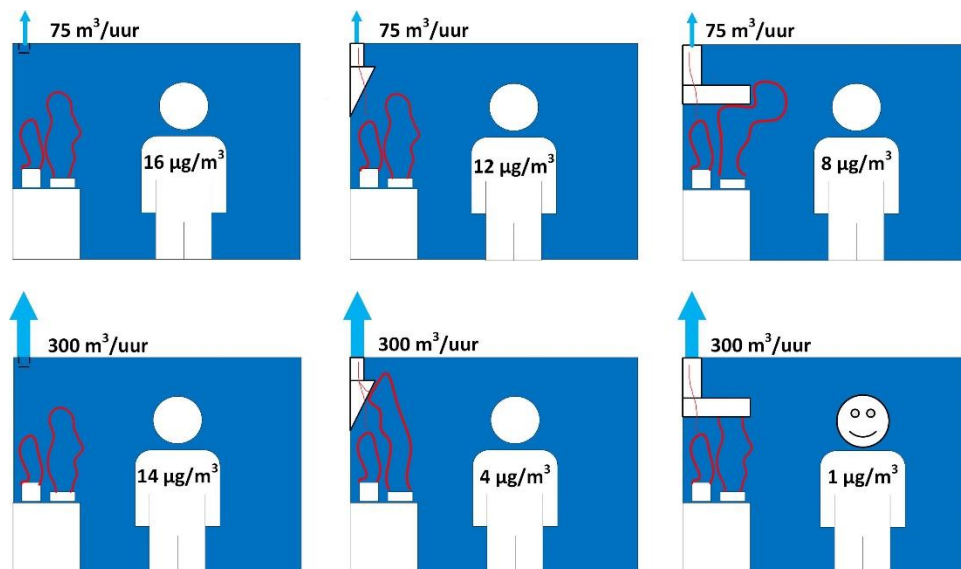
Figuur 7 jaargemiddelde PM 2,5 concentratie verhoging bij verblijf in woning door koken.
